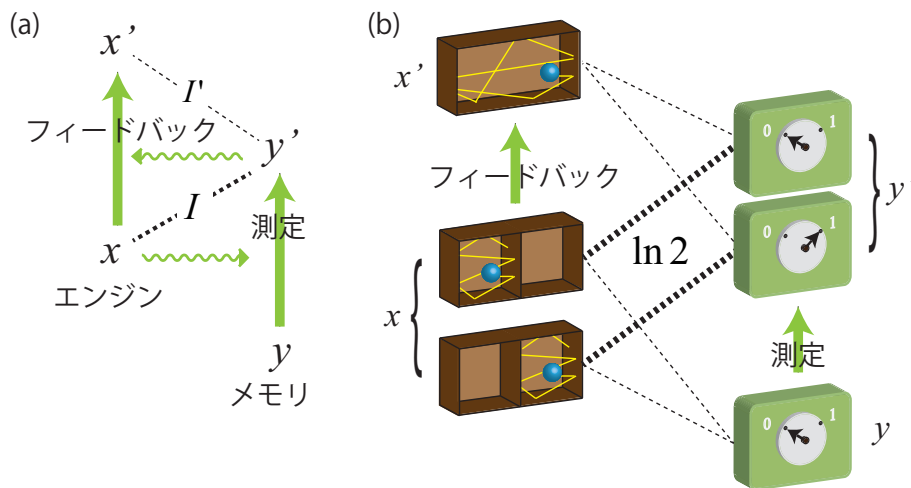
図 5: 測定とフィードバックの模式図。(a) 一般的な設定。まず測定するとき、エンジンの被測定状態 x の影響を受けながら、メモリの状態が y から y' まで変化する。この間は x は変化しないとする。測定後の x と y' の相関が、メモリが測定で得た情報に対応する。次にフィードバックによって、メモリの測定結果 y' の影響を受けながら、エンジンの状態が x から x' まで変化する。この間は y は変化しないとする。(b) シラード・エンジンの場合。
